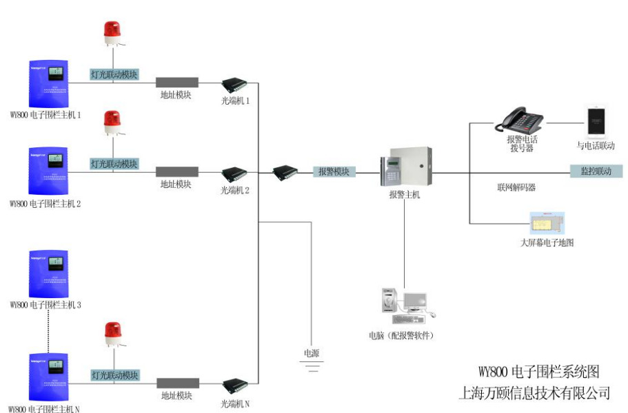
典型电子围栏组网系统图
